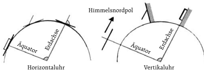
Abb. 11: Horizontal- und Vertikaluhr: Die Zeigerwinkel sind erdachsparell
