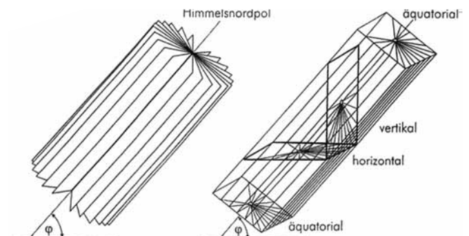
Abb. 10: Konstruktionsschema für verschiedene Zifferblattarten
