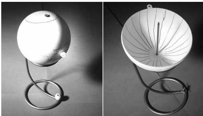
Abb. 19, 20: Skaphe (Hohlflächensonnenuhr, Plexiglas): Beim Transport wird die Kompassnadel in der verschlossenen Kugel verstaut, bei der Zeitmessung anstelle der abnehmbaren Holzkugel am Fuß angebracht.
