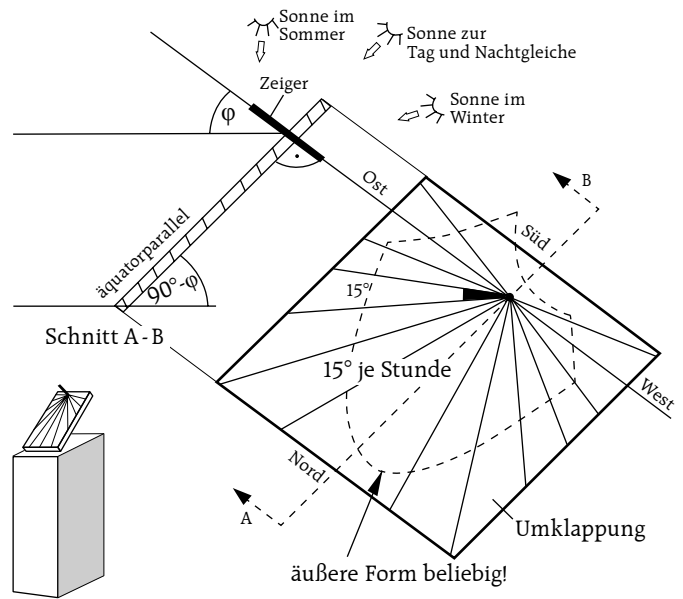
Abb. 9: Äquatorparalleles Zifferblatt: Typische Auffächerung der Stundenlinien
