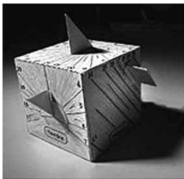
Abb. 11: Horizontal- und Vertikaluhr: Die Zeigerwinkel sind erdachsparell
