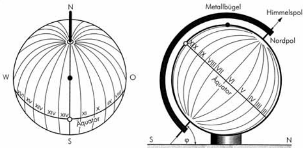
Abb. 6: Kugel- und Globussonnenuhr
