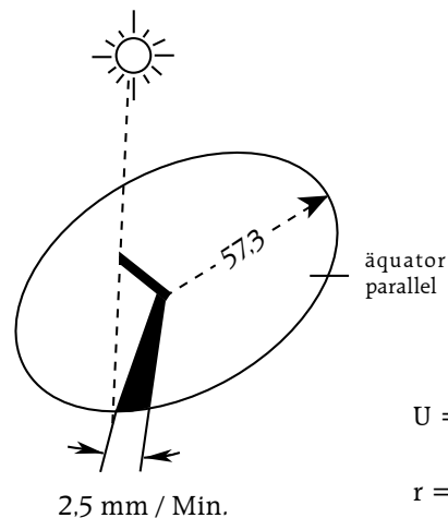
Abb. 4: Wanderweg des Schattens: Der Schatten wandert bei einer äquatorialen Sonnenuhr pro Stunde um 15^\circ . Auf einem Kreis von 360 cm Umfang wandert er mit 2,5 mm/Minute
