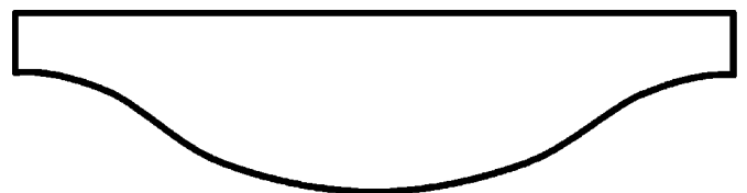
Abb. 8a: Lehre zur Bildung der Grundform der "Chaosschüssel"
