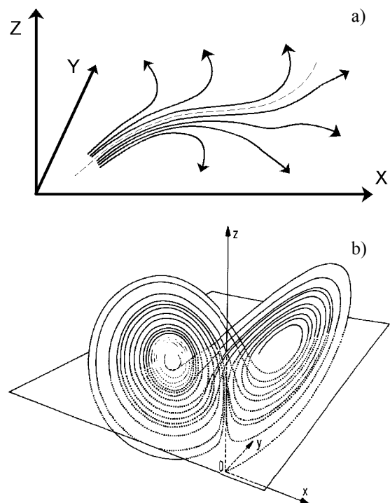
Abb. 2: Dynamische Instabilität (a) und strukturelle Stabilität (b) chaotischer Systeme
