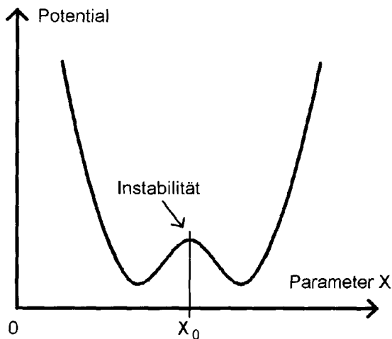
Abb. 3: Prinzipieller Potentialverlauf bei chaotischen Systemen
