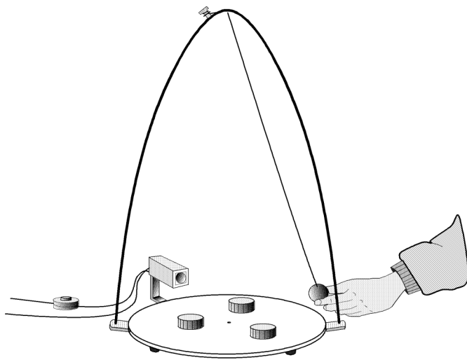
Abb. 5: Schematischer Aufbau des Magnetpendels
